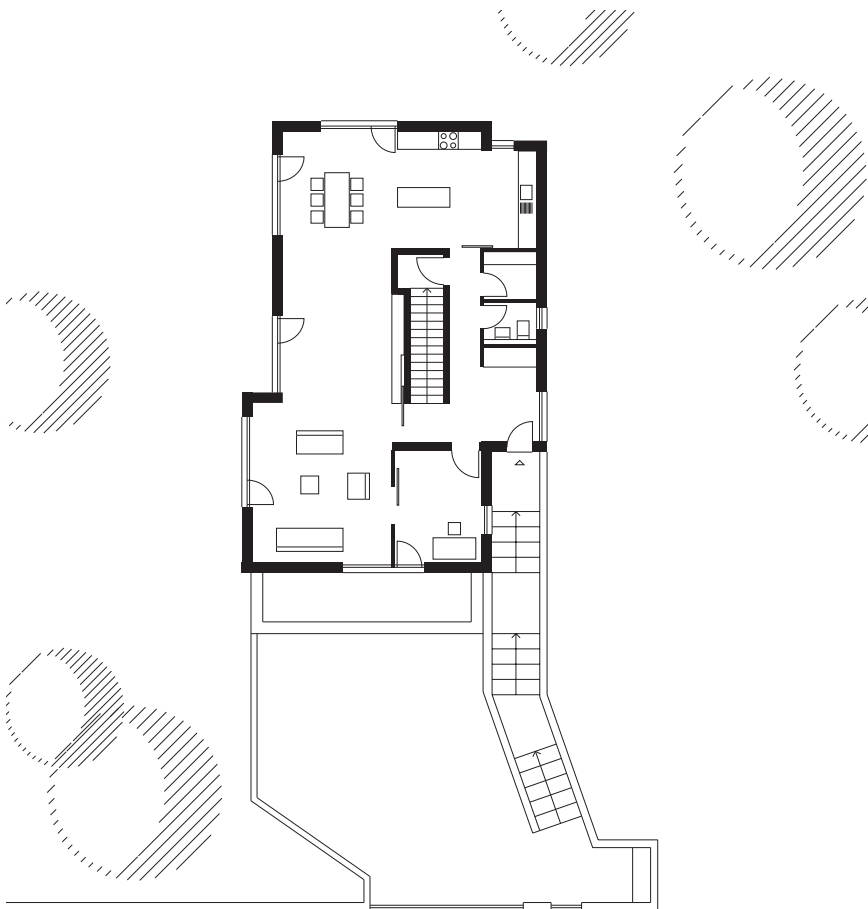
Grundriss EG
