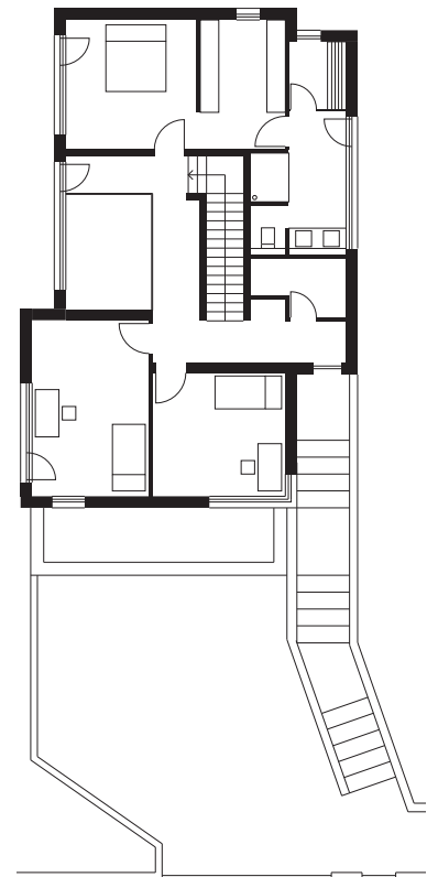
Grundriss OG
